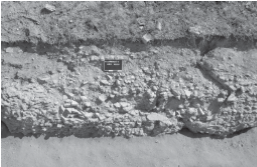
Fig. 6 - Particolare della struttura, con tracce riferibili ad una vasca.
